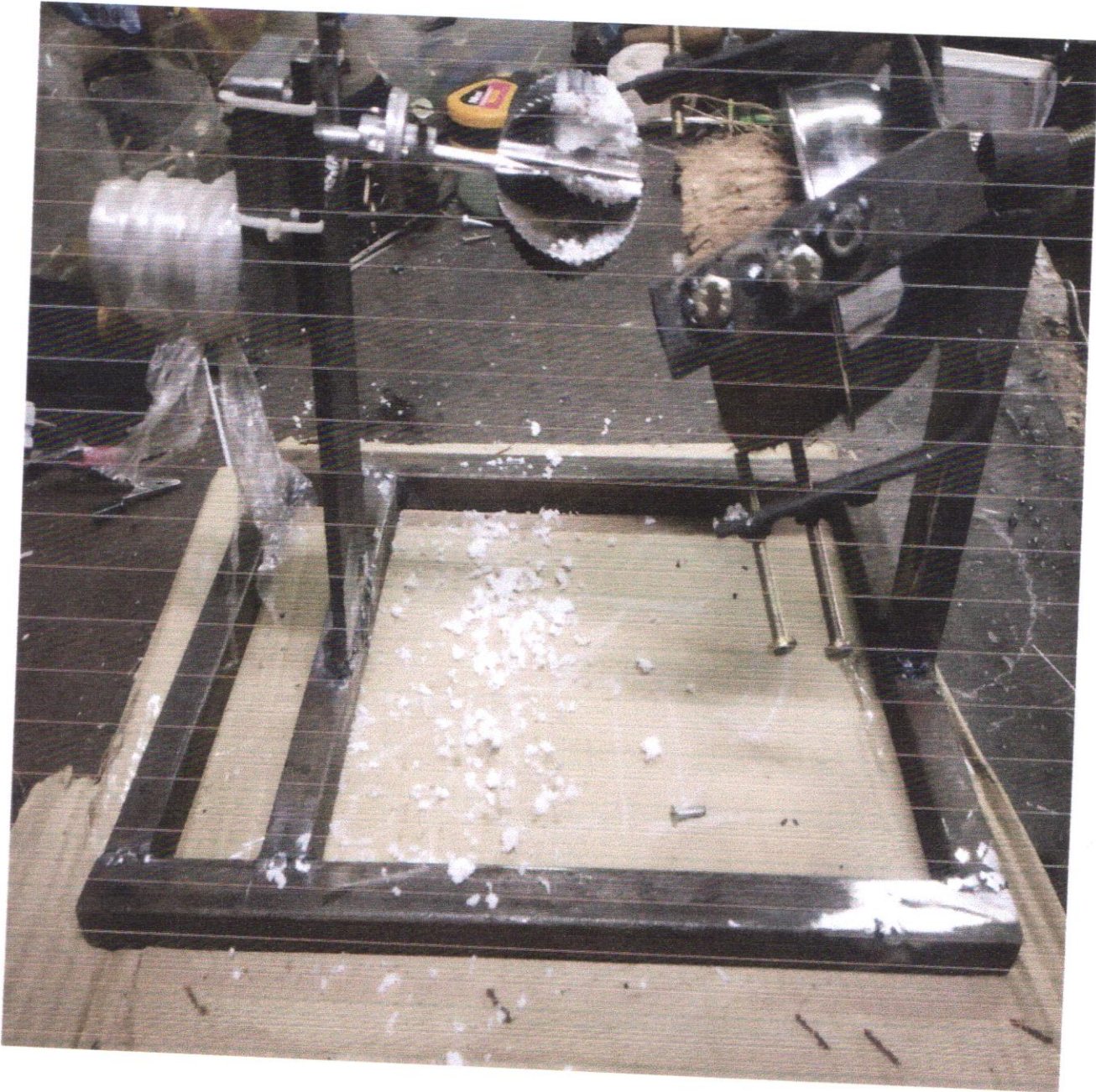
mini coconut scraping machine
